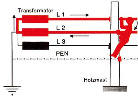
Bild 2-5: Stromfluss bei der Berührung von zwei Außenleitern
